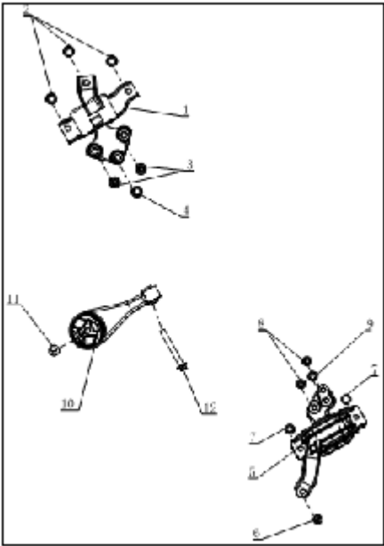
发动机安装分解图(搭载SFG18+CVT发动机)
