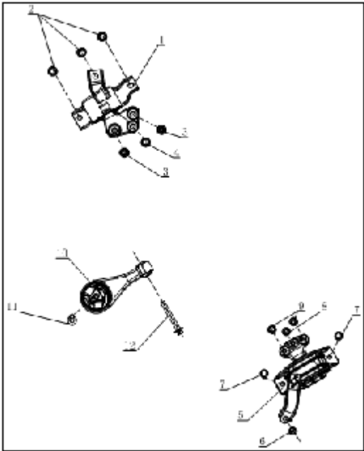
发动机安装分解图(搭载SFG15T+6MT汽油发动机)
